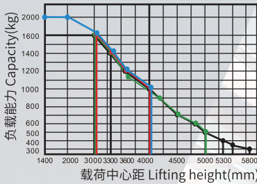
载荷曲线图 Load curve
